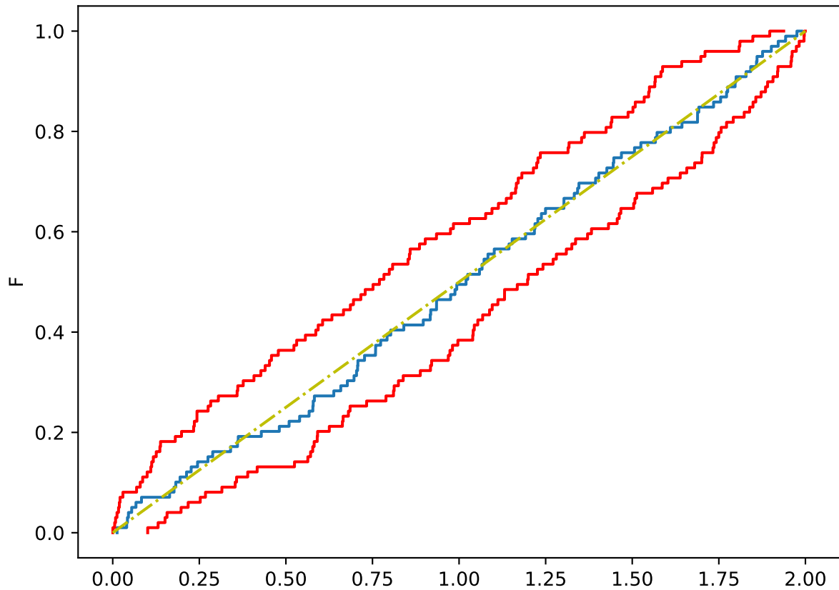
emp. Verteilungsfunktion mit MC-Bändern
